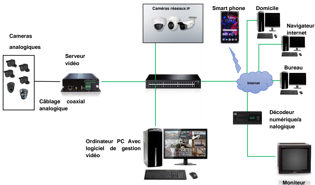
Figure 2 : schéma synoptique du principe de fonctionnement de la vidéosurveillance sur IP
